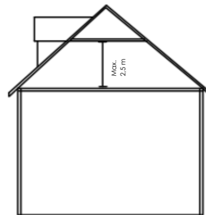
Giebelgauben
