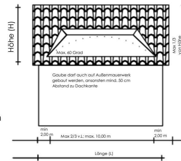
Schleppgauben
