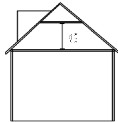
Flachdach-Gauben
