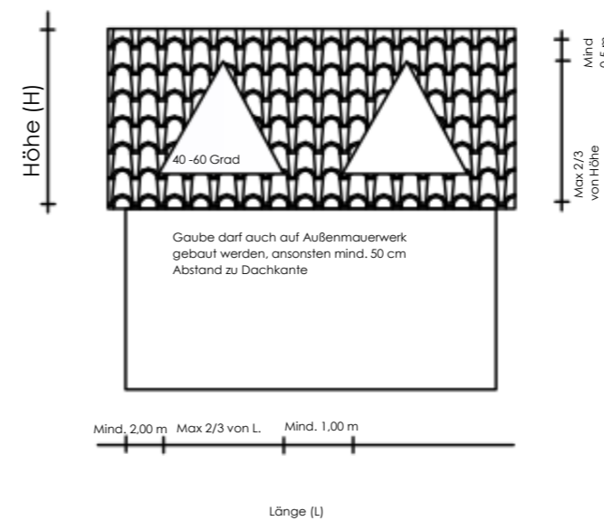
Giebelgauben
